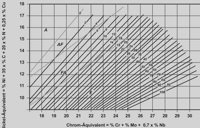
WRC - 92 - Diagramm (nach D. J. Kotecki und T. A. Siewert, Welding Journal; Mai 1992, Seite 171-s bis 178-s)
