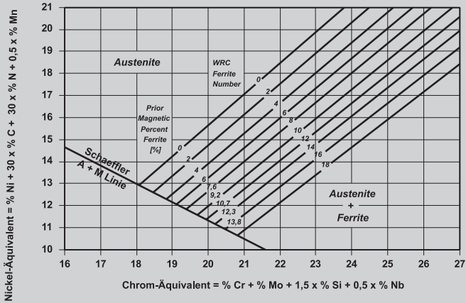
DeLong - Diagramm (nach W. T. DeLong, Welding Journal, Juli 1974, Seite 273-s bis 286-s)
