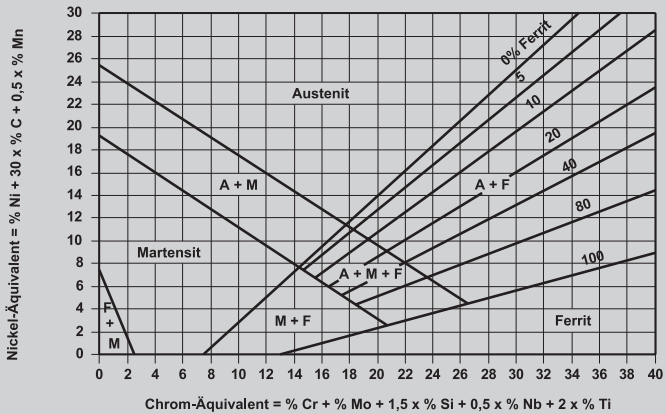
Schaeffler - Diagramm (nach A. L. Schaeffler, Metal Progress Nov. 1949, Seite 680 bis 680-B)
