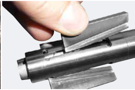
Das Spannsystem "NC" ist mit seinen im Mast fest verankerten Spannkeilen unverlierbar
